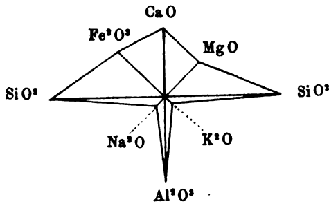
Fig. 5. Rizzonit, Schlucht zwischen Ricoletta und Rizzoni (Südseite) (DOELTER analys.) 3 .
